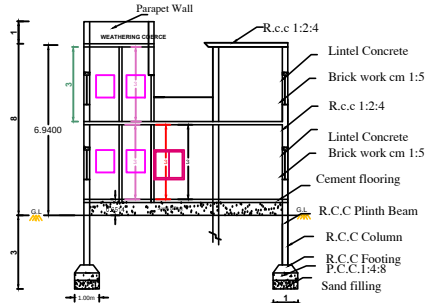
SECTION - AB
