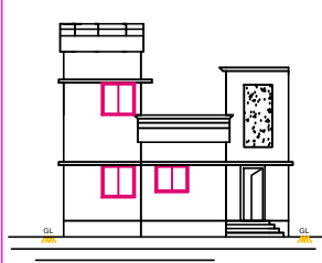
ELEVATION
