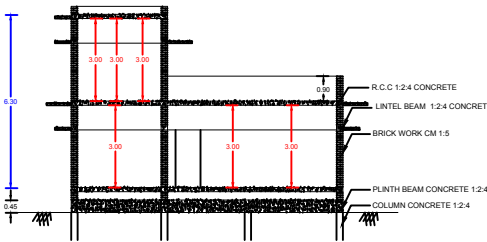
SECTION A-B
