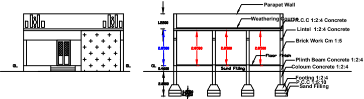
Elevation
