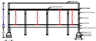
SECTION - AB
