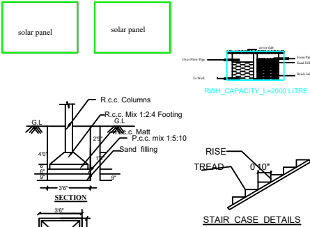
R.C.C. COLUMNS DETAILS
