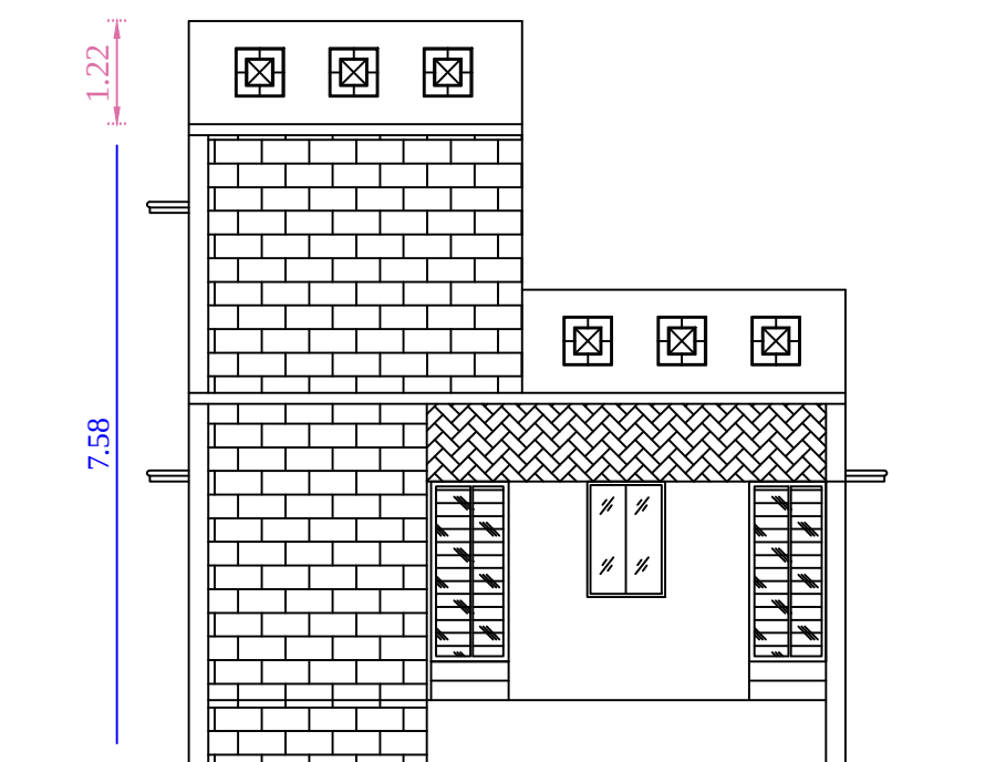
ELEVATION
