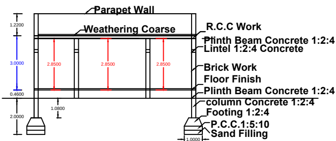
SECTION - AB
