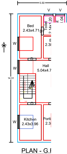
PLAN - G.I
