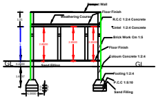
Section - AB
