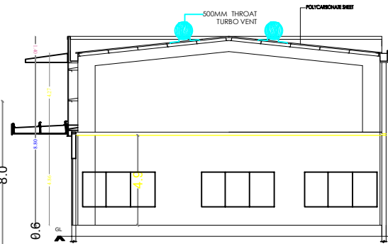
SECTION A-B
