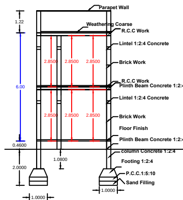
SECTION - AB
