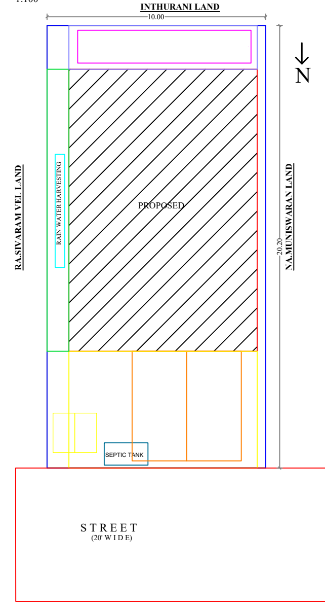
SITE PLAN 1:100
