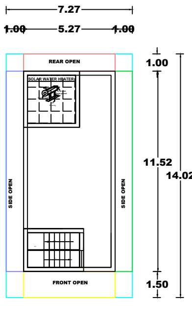
Open Teracce
