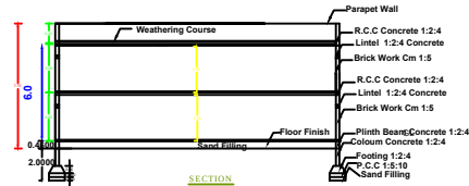
SECTION - AB
