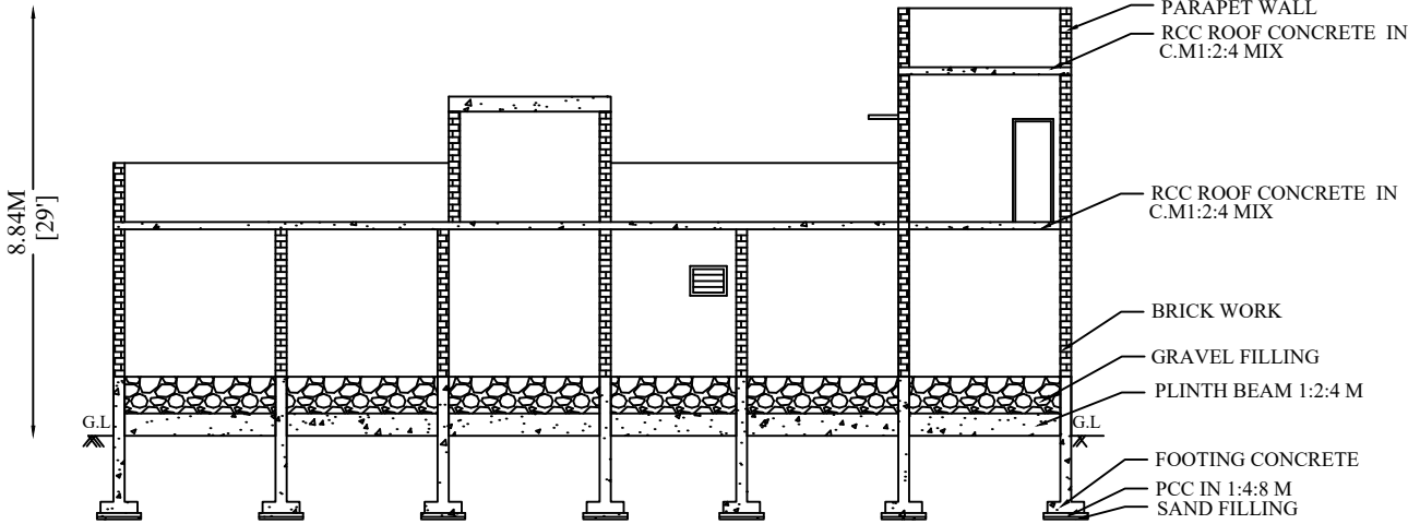
SECTION A-B
