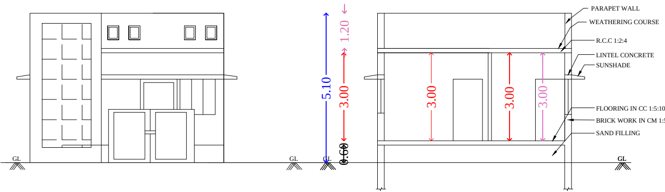
ELEVATION
