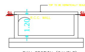
RW1 SECTION (SAMPLE)
