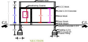
SECTION - AB
