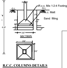
R.C.C. COLUMNS DETAILS
