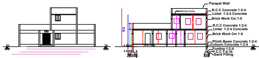
Elevation
