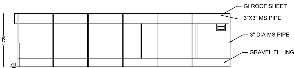
SECTION A-B
