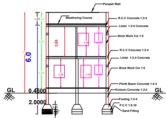
SECTION - AB
