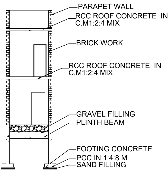
SECTION A-B
