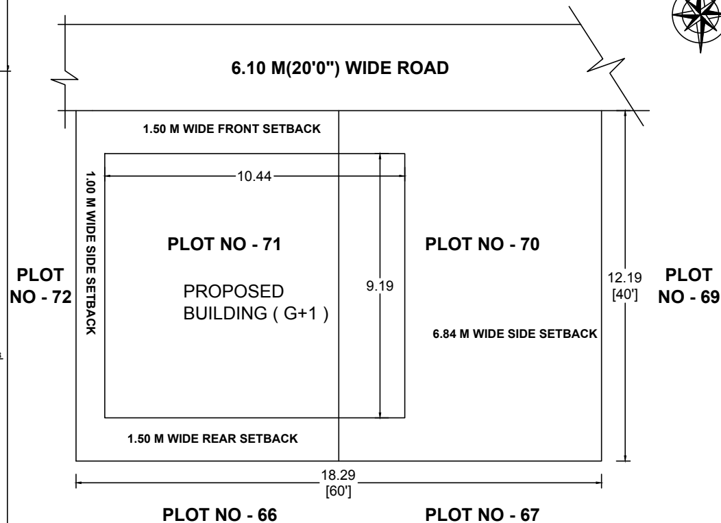
SITE PLAN :
