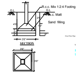
R.C.C. COLUMNS DETAILS
