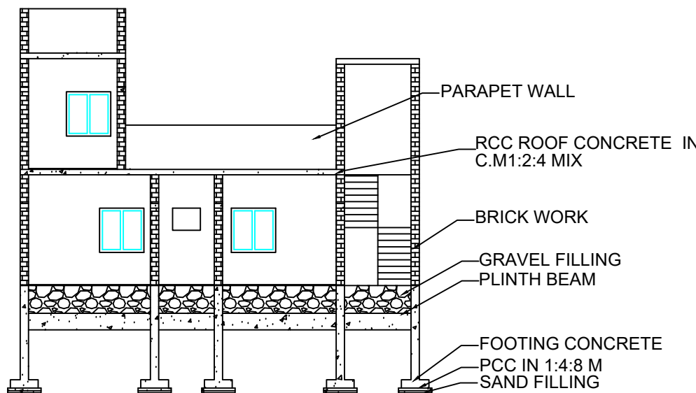
SECTION A-B
