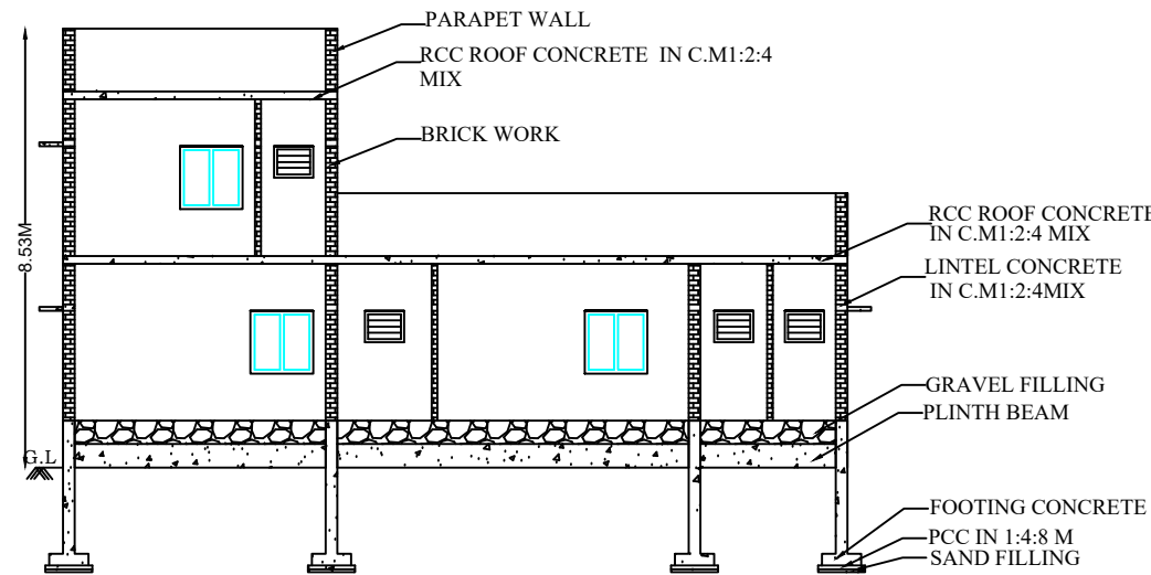
SECTION A-B
