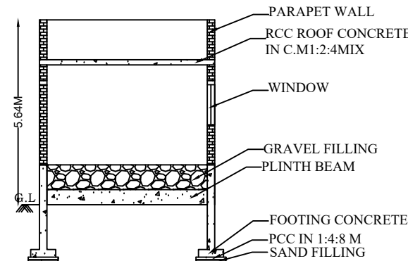
SECTION C-D
