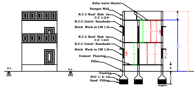
Elevation
