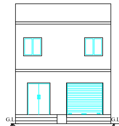
ELEVATION
