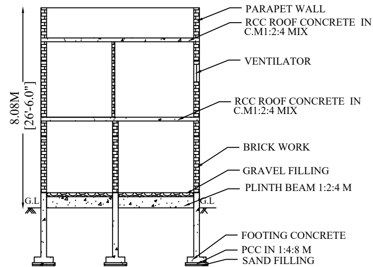
SECTION A-B
