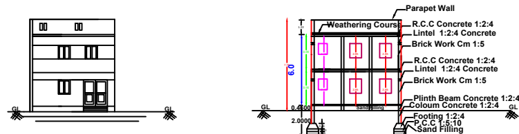
Elevation
