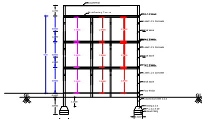
SECTION - AB
