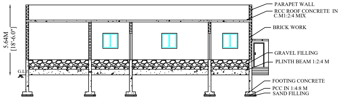
SECTION A-B
