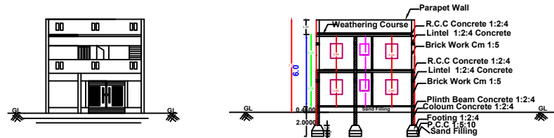
SECTION - AB
