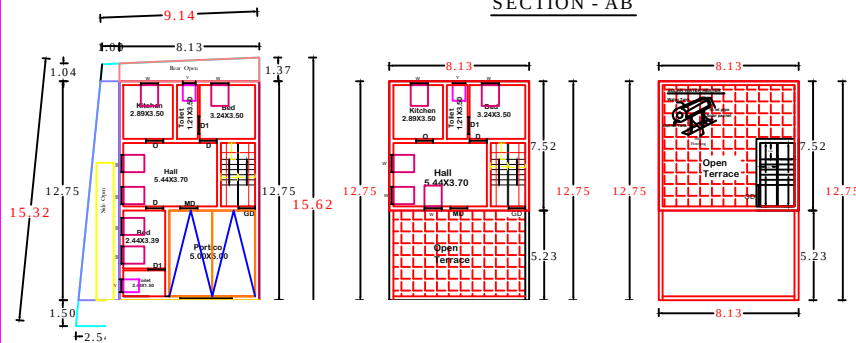
SECTION - AB
