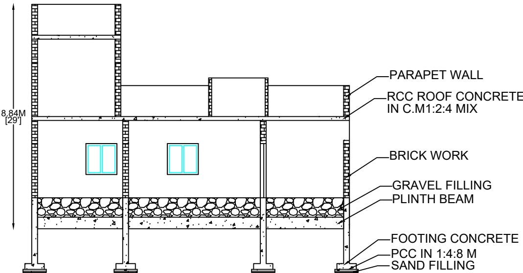
SECTION A-B
