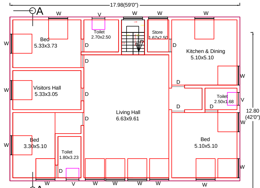
PLAN - F.F
