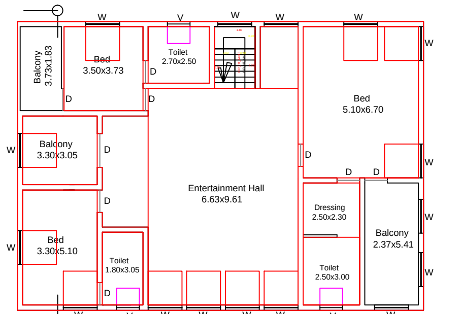
PLAN - S.F
