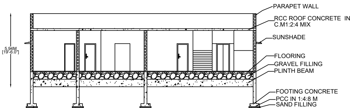
SECTION A-B
