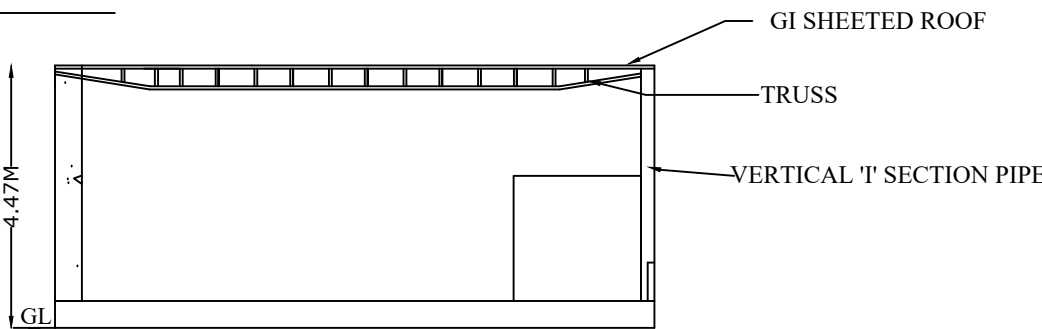
SECTION A-B
