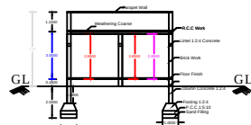
SECTION - AB
