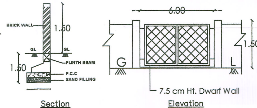
Elevation
