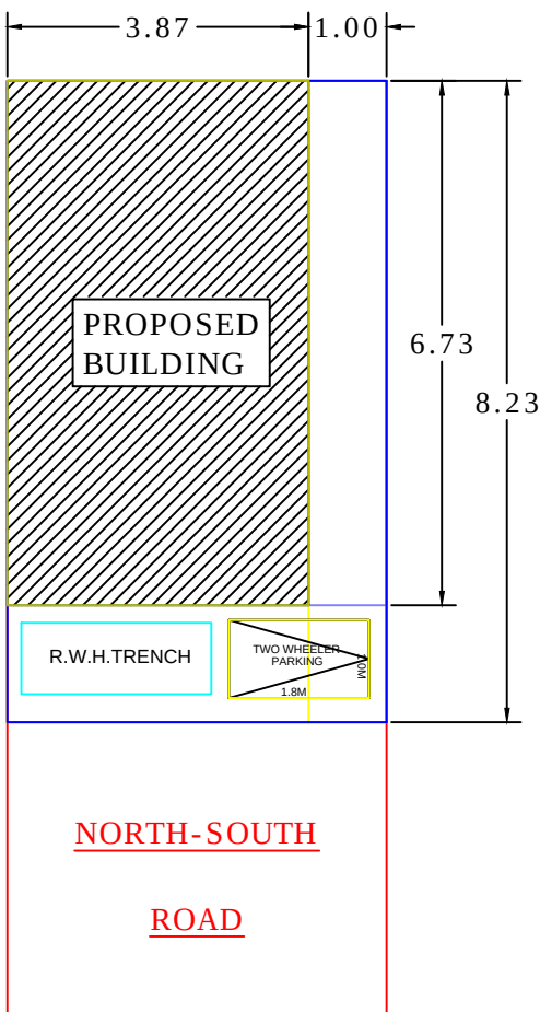
SITE PLAN BALANCE 320 SQ.FT LAND
