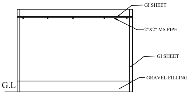
SECTION A-B
