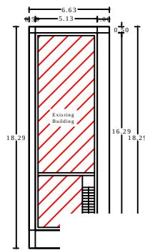
Groun
