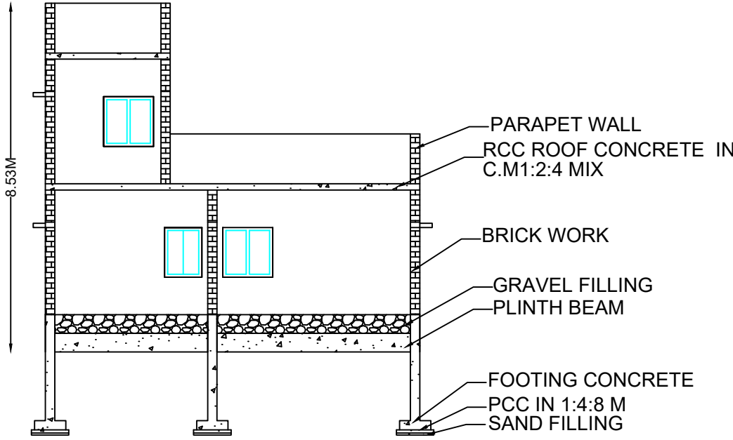
SECTION A-B
