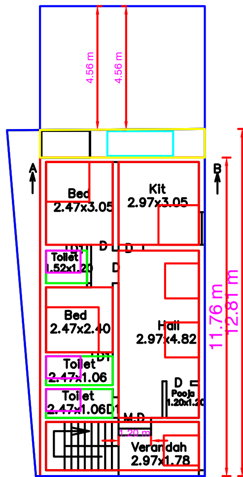
Firstfloor(Pro.)
