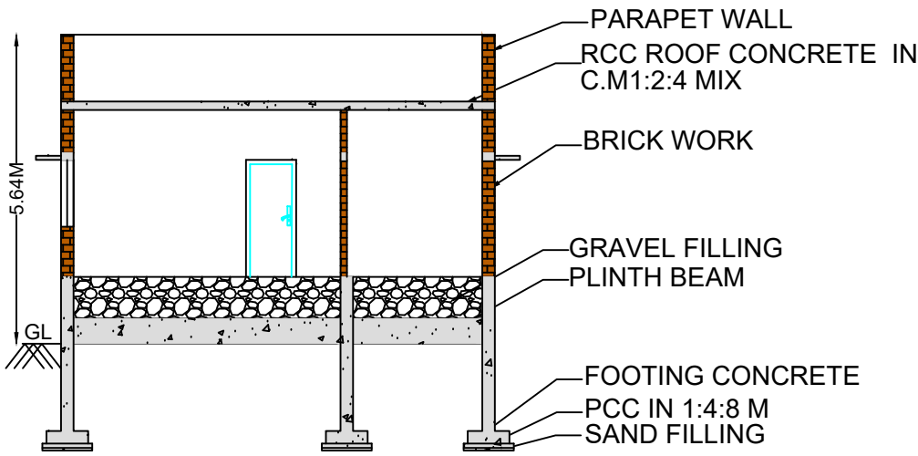
SECTION A-B
