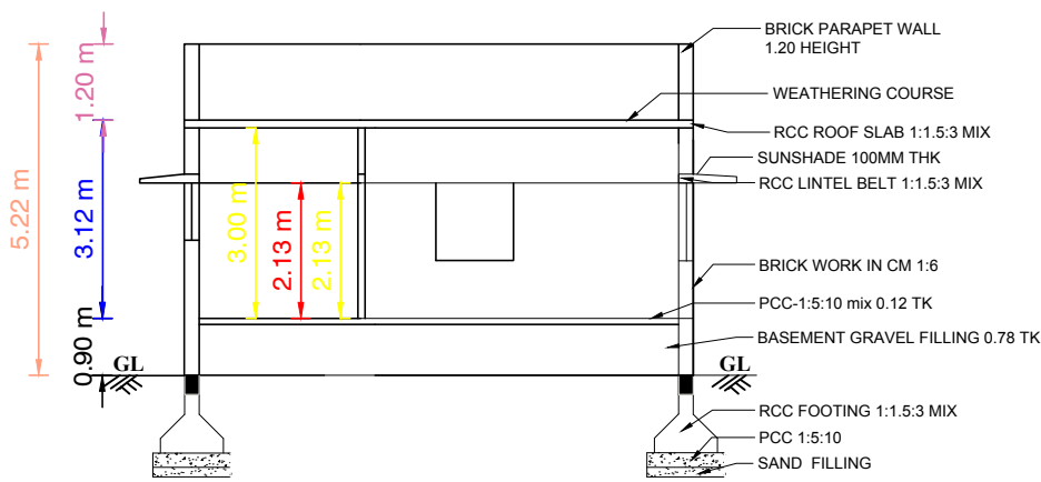
SECTION A-A
