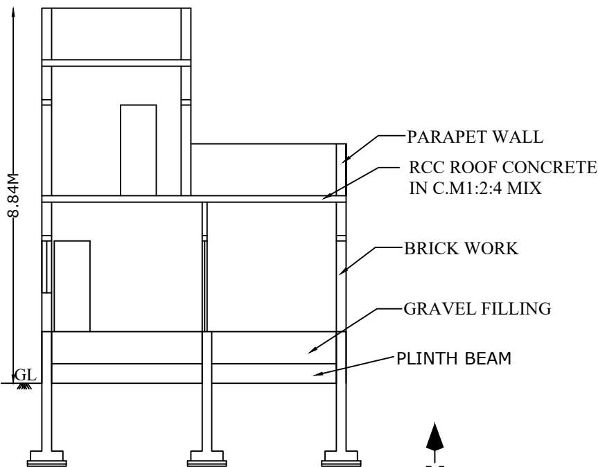
SECTION A-B
