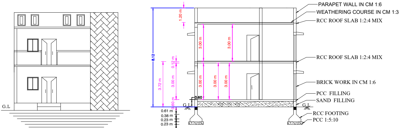
ELEVATION
