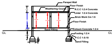
SECTION - AB
