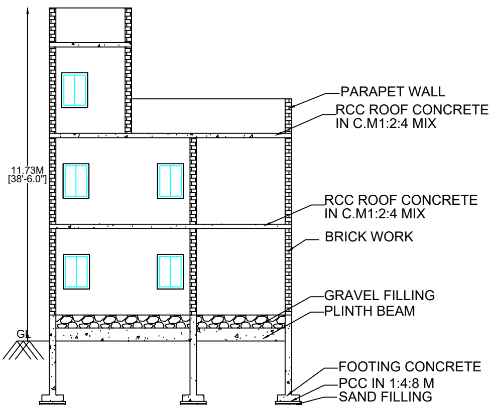
SECTION A-B
